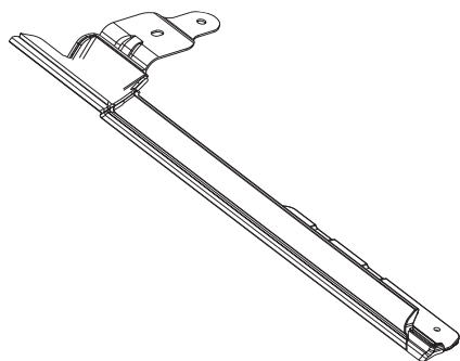
Rail de porte - Supérieur gauche Pièce n°597.03 Qté. 1
