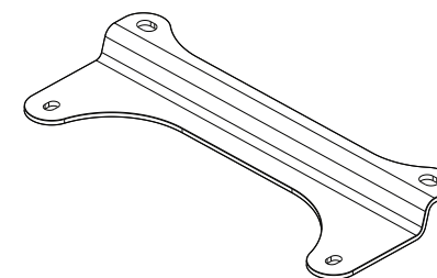
Support, Attache centrale Halo Pièce n°597.18 Qté. 1
